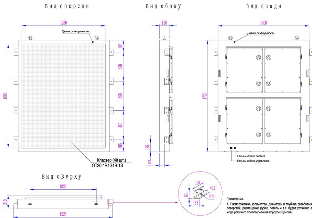
Рис. 2. Внешний вид и основные размеры ДЗПИ.
