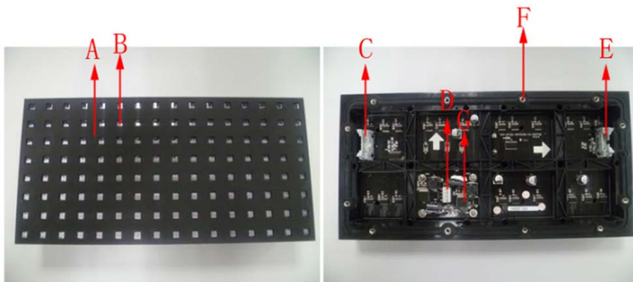
Рис.1 Кластер УНТ-FVMS-OT20-1R1G1B-1S. Лицевая поверхность и тыльная сторона.
