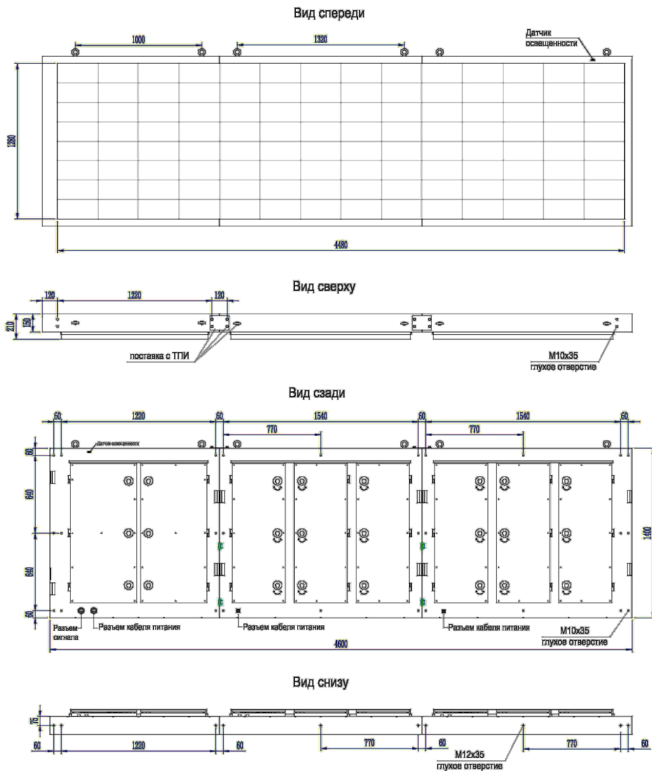
Рис. 3. Внешний вид и основные размеры ДИТ.
