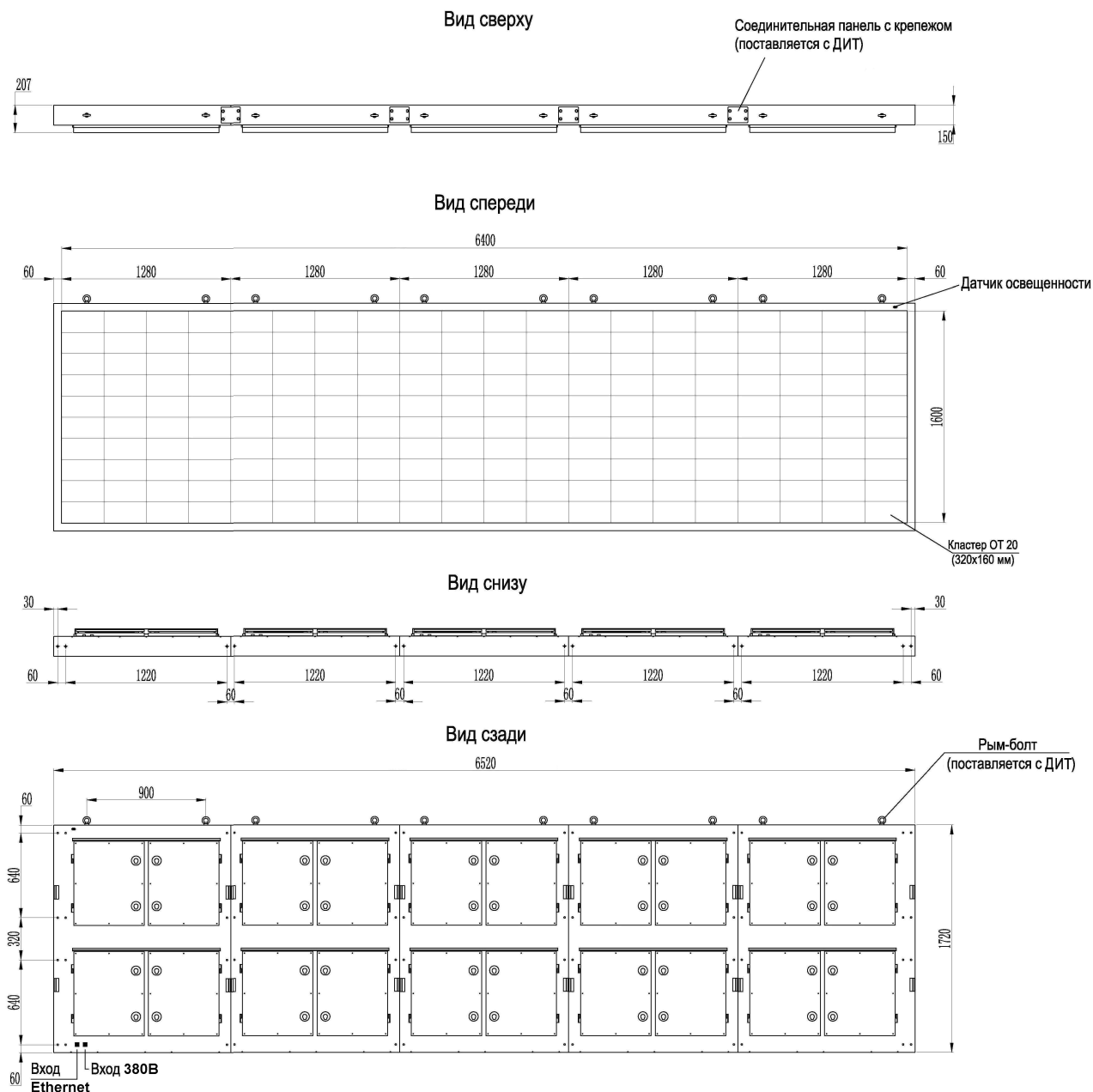
Рис. 2. Внешний вид и основные размеры ДИТ.
